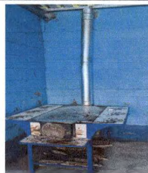
Foto 2: Implementación de estufa rural completa incluye chimenea y plancha de metal
