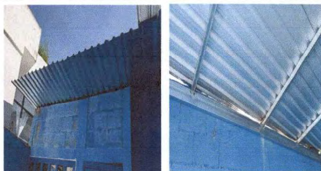
Foto 10: Implementación de lámina troquelada Aluzinc calibre 26 y estructura de soporte de metal para techo.
